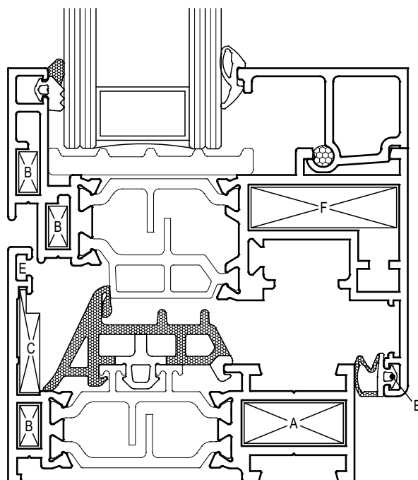
TS205 SQUADRETTA A SPINO - CIANFRINARE
